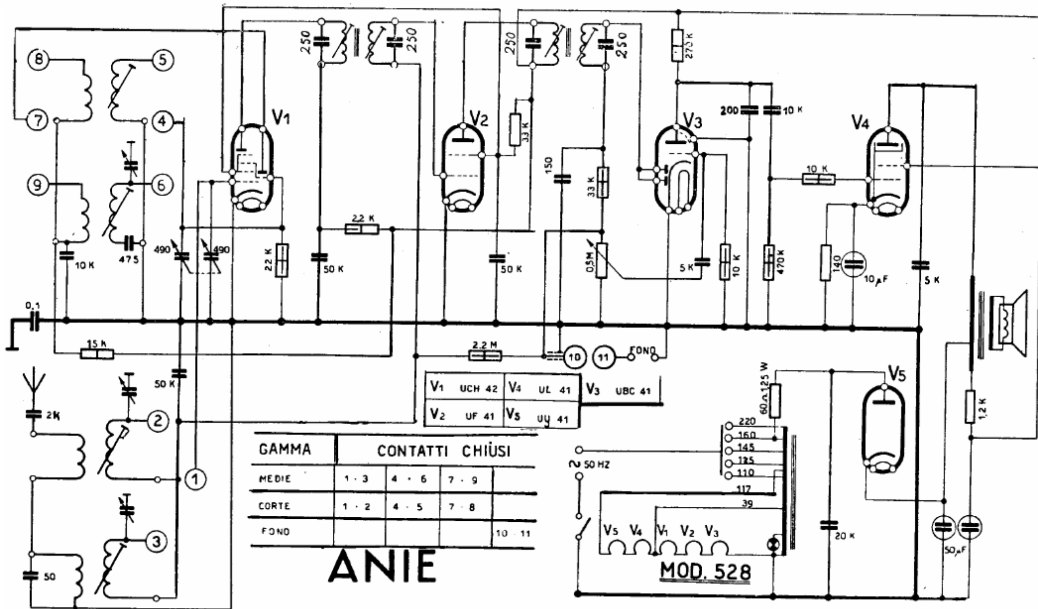
VEGA - Mod. 528. Serie ANIE. Onde medie da 520 a 1620 kc/s. Onde corte da 5,8 a 18 Mc/s. Punti di taratura 580-1500 kc/s. Media frequenza 470 kc/s. Potenza indistorta di uscita 2,5 watt. Consumo 42 watt.
